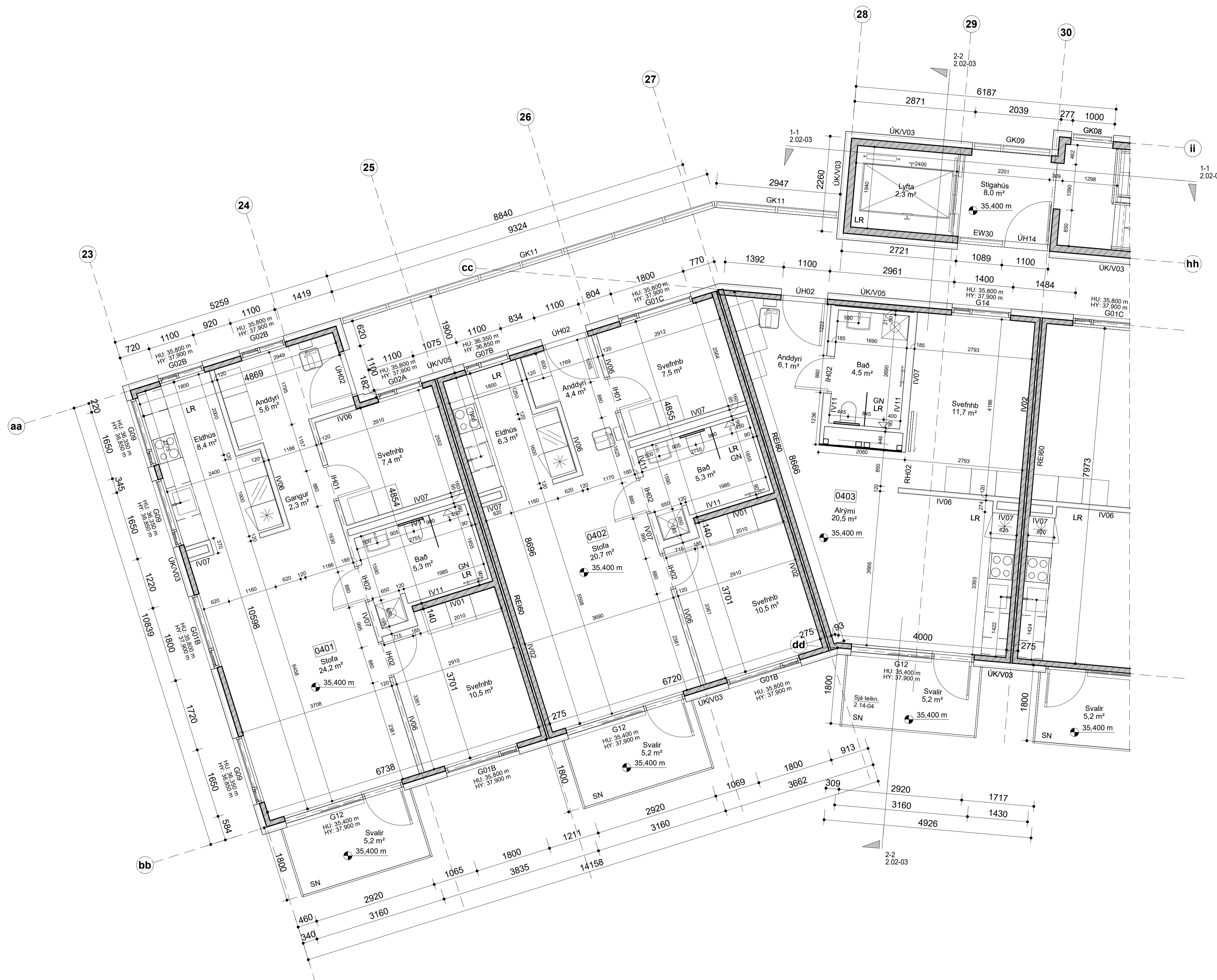
4.hæð- Verk. hús 8 - hluti 1/2 mkv: 1 : 50
