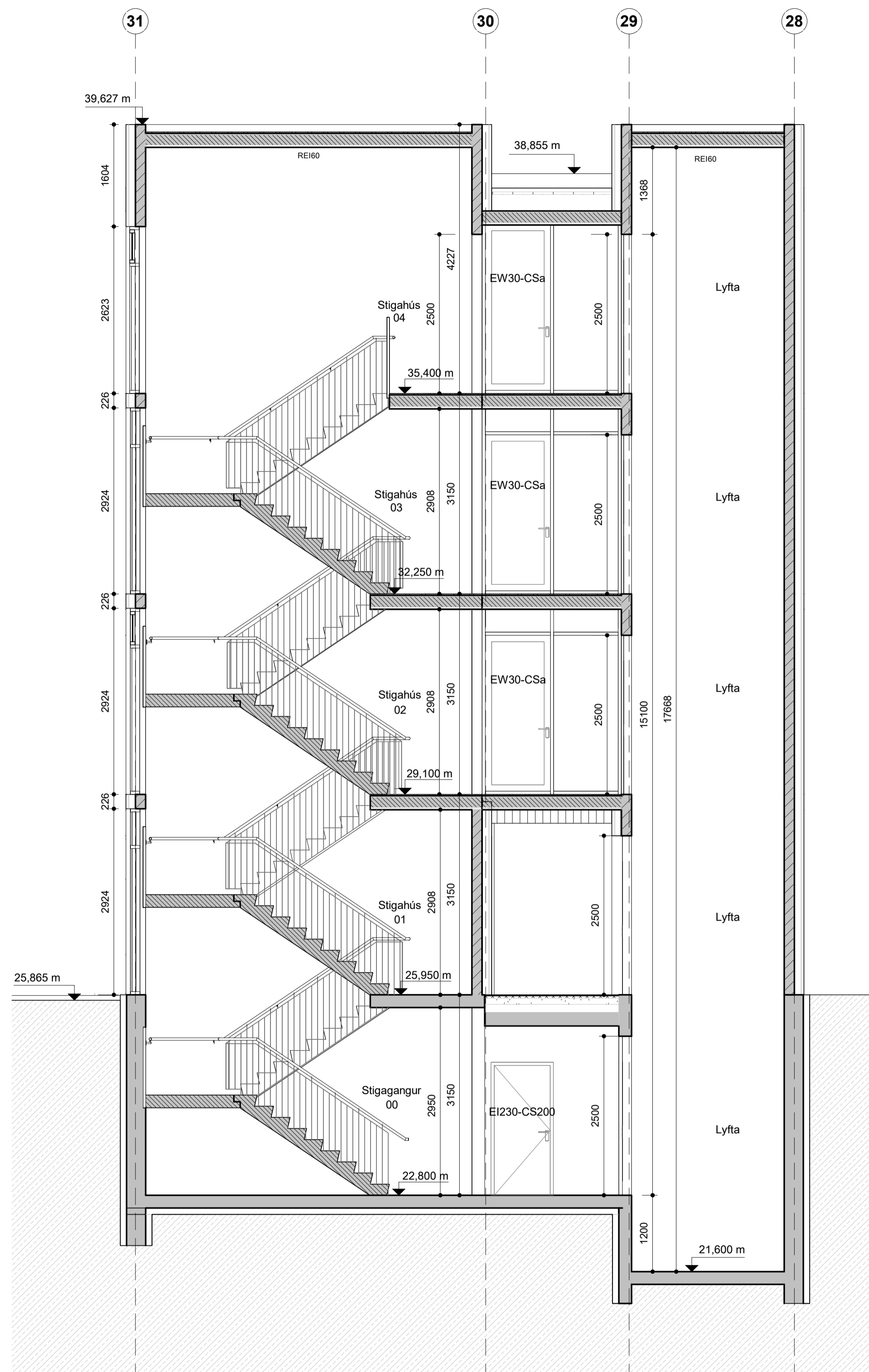
Hús nr 8 - Snið 1, verkt. mkv: 1 : 50
