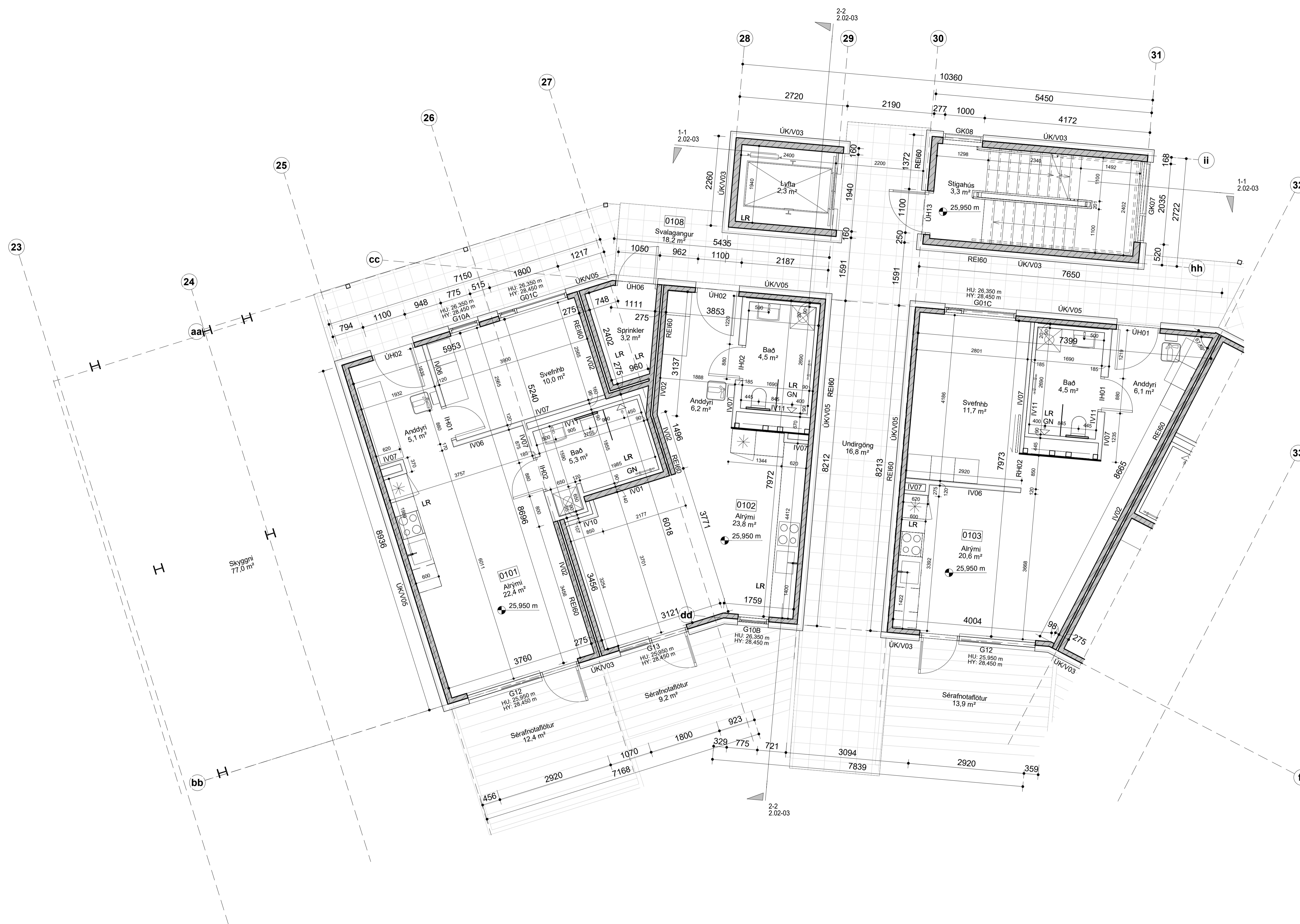
1.hæð hús 8- verk. hluti 1/2 mkv: 1 : 50
