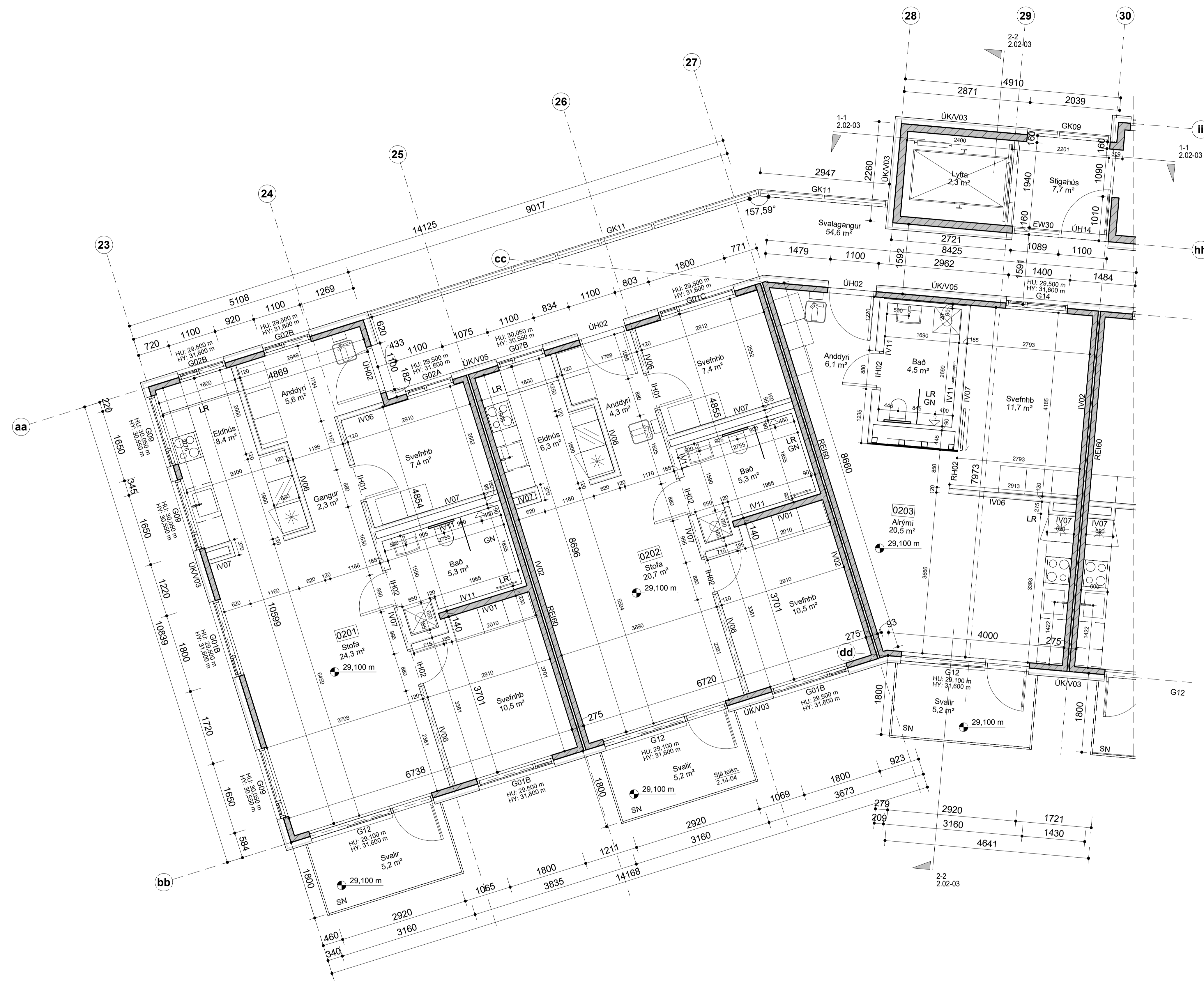
2.hæð - Verk. hús 8 - hluti 1/2 mkv: 1 : 50
