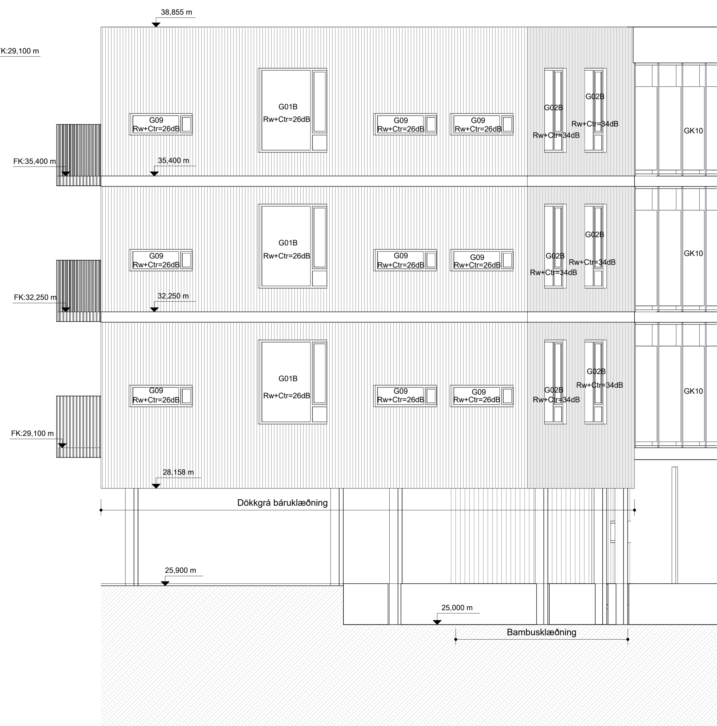
Austur - Verk, hús 8 mkv: 1 : 50
