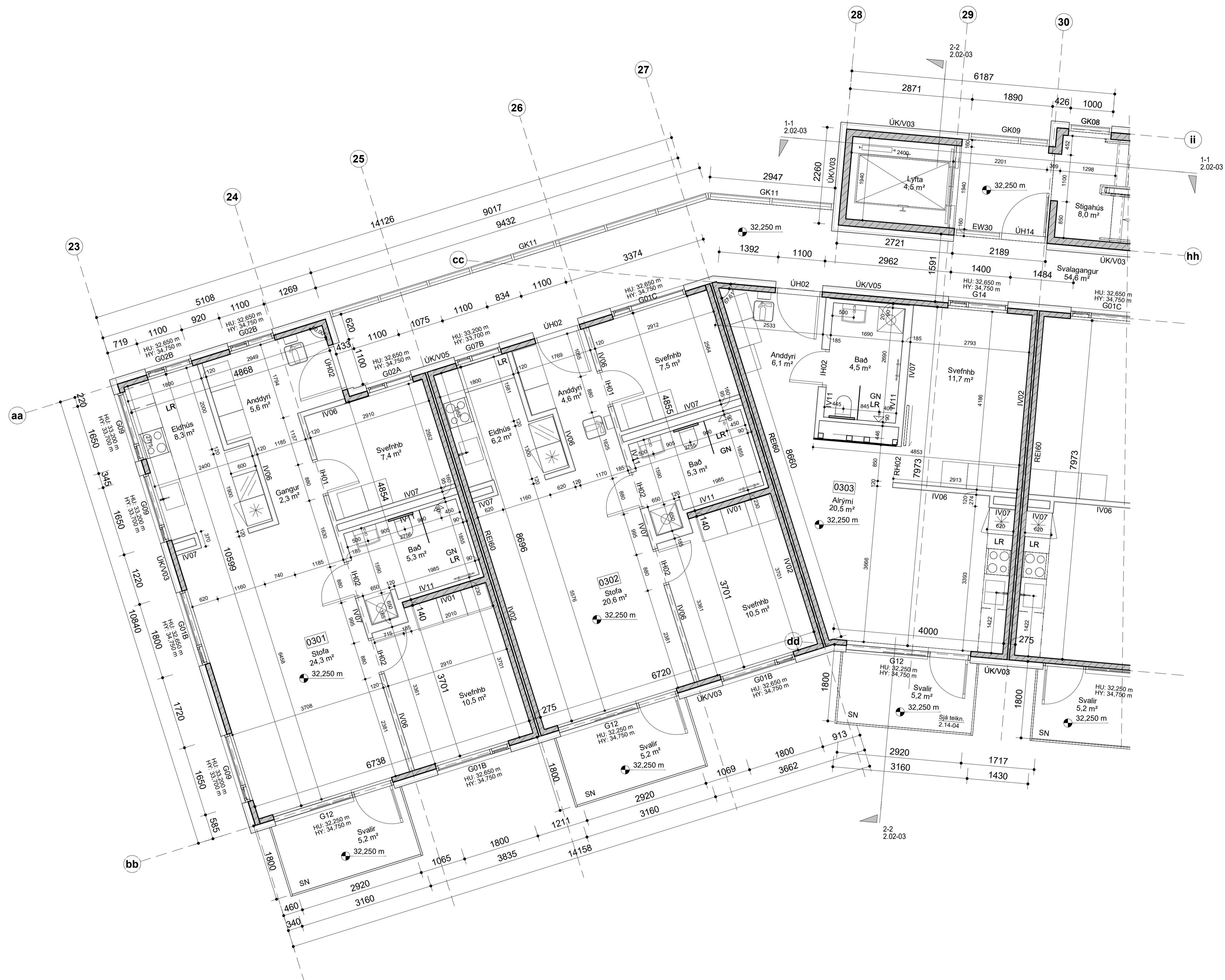
3.hæð - Verk. hús 8 - hluti 1/2 mkv: 1 : 50
